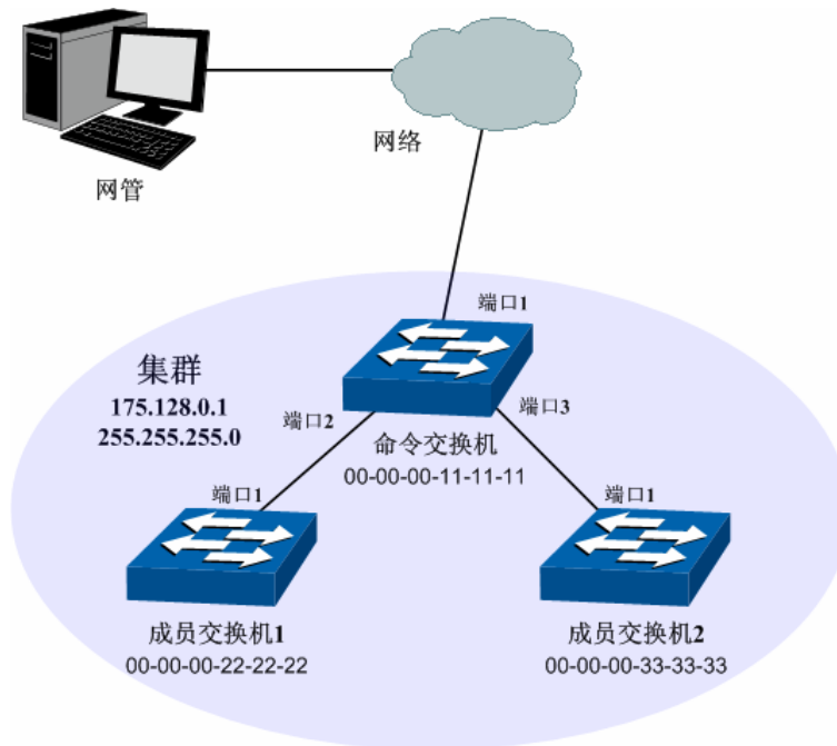
图 14-15 集群管理组网图
