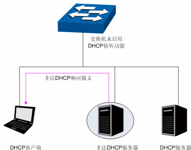
图 11-7 DHCP服务欺骗攻击
