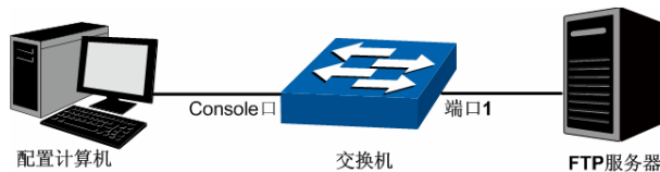
图 16-1 利用FTP加载软件连接图
