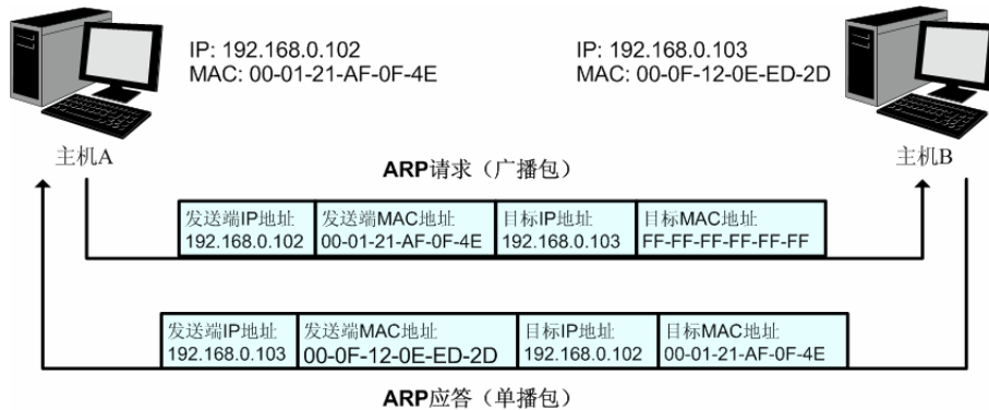
图 11-3 ARP地址解析图
