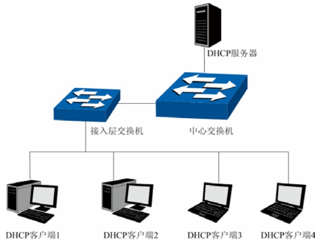
图 11-5 DHCP网络典型应用
