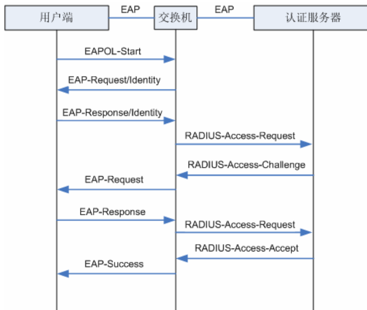
图 11-18 EAP-MD5认证过程
