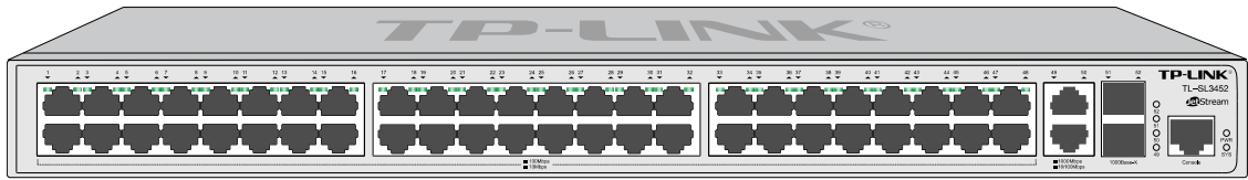
图 2-2 TL-SL3452前面板
