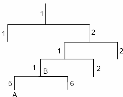
图 12-2 MIB树结构
